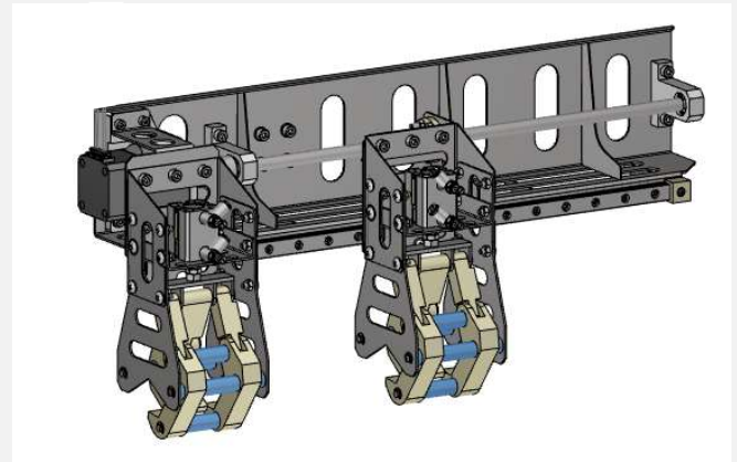
例) 把持ピッチ調整機構付きハンド
