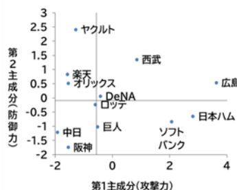
主成分分析：散布図
